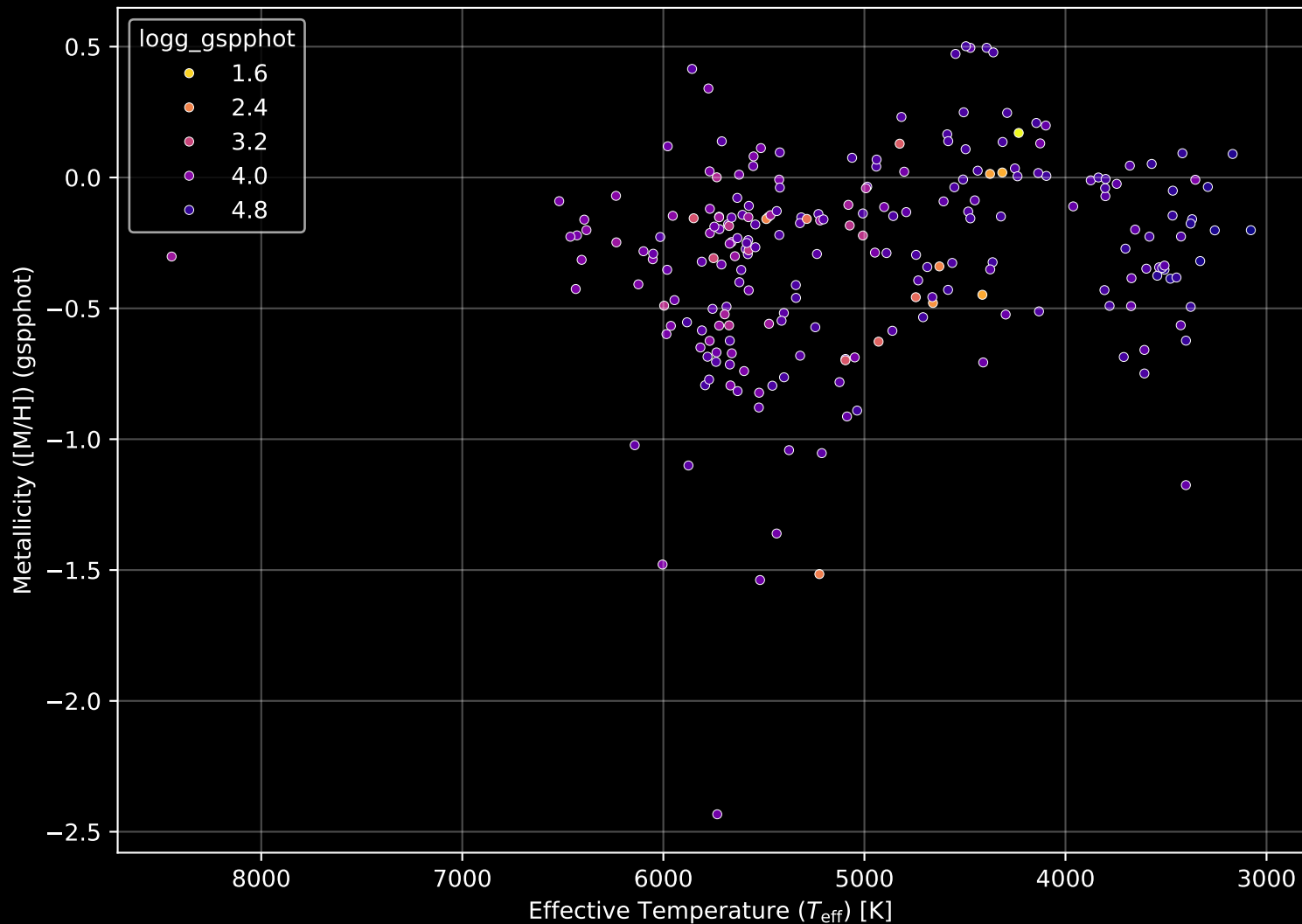
APOGEE DR17 Field: [Sgr_tidal3] Stellar Population Parameters (n= 230)
